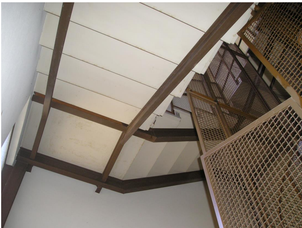
13. La struttura metallica di protezione antisismica in uno dei vani scala
