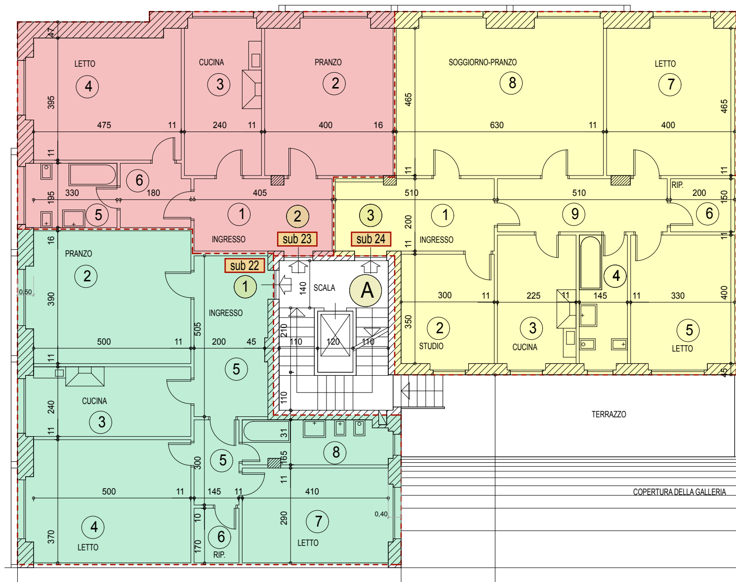
Piano PRIMO
