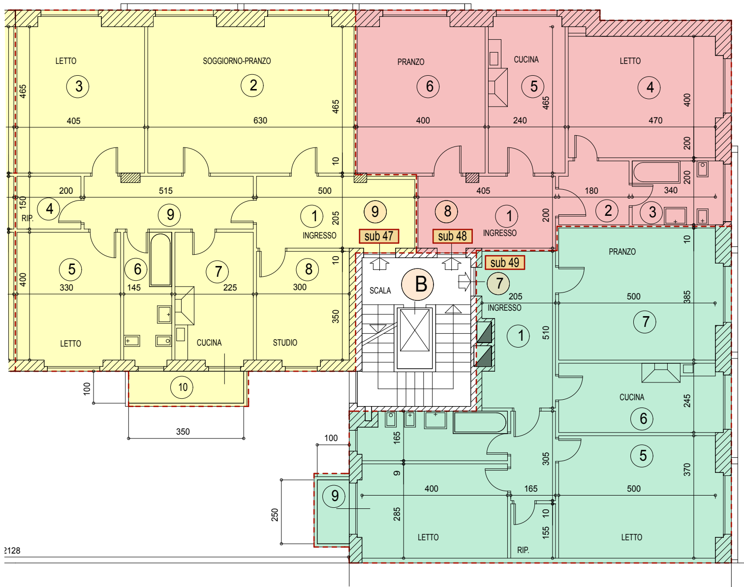
Piano TERZO
