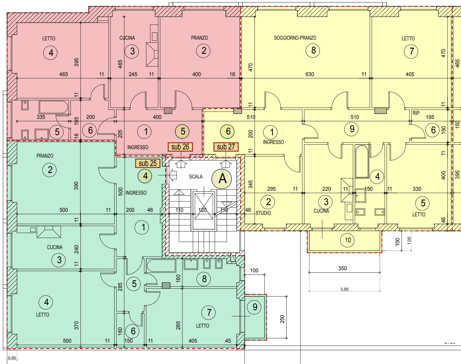
Piano SECONDO
