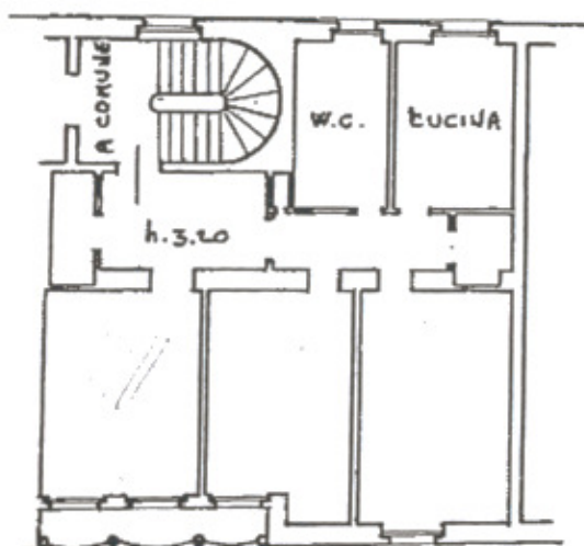
PIANO TERZO
